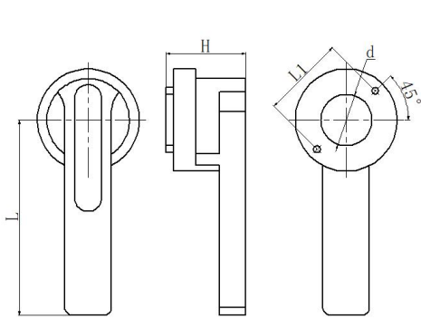
B2 B3型
