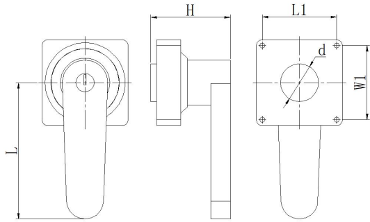
H 型带锁
